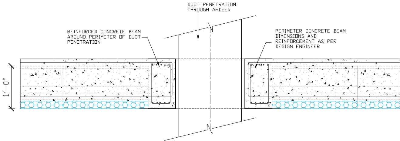
LONGITUDINAL SECTION
